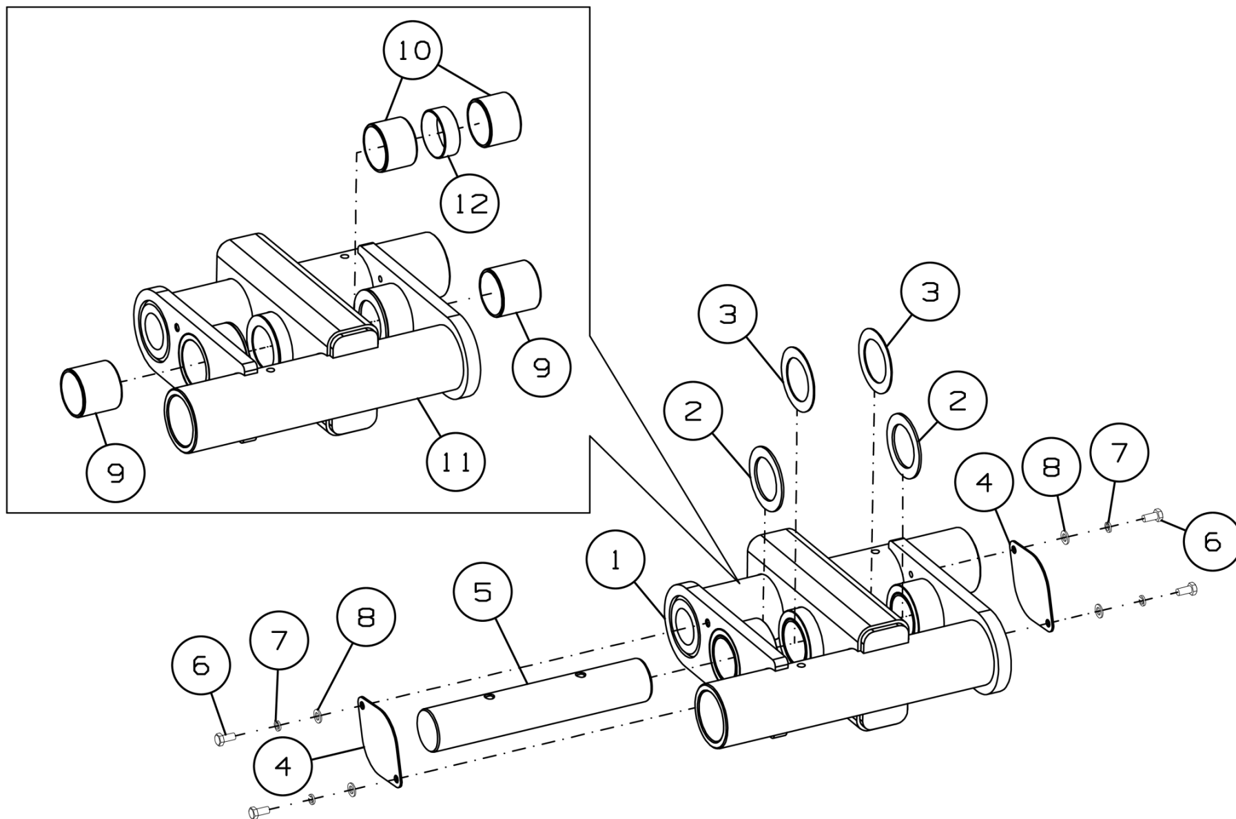
Рисунок 25 - Балансир в сборе ДХ-1080.08.100Б
