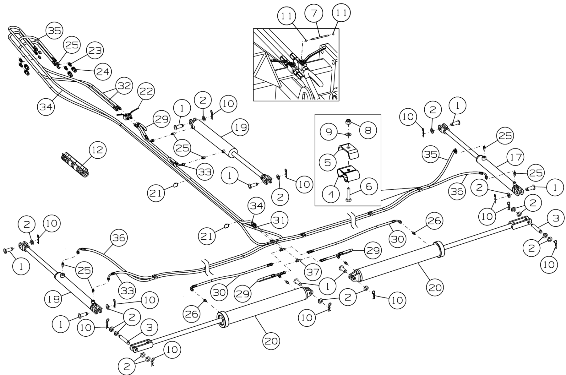
Рисунок 28 - Установка гидрооборудования ДХ-1080.12.000А
