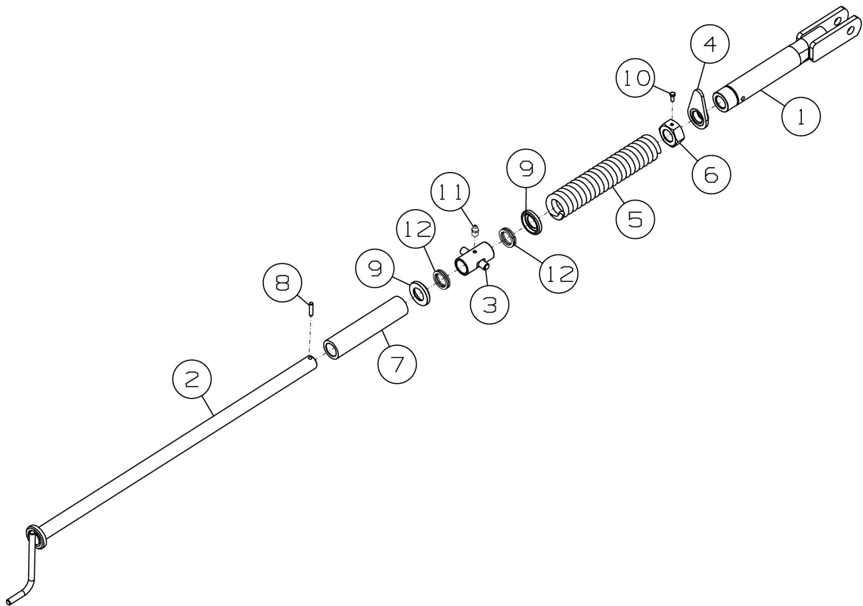
Рисунок 21 - Регулятор горизонта ДХ-1080.05.100
