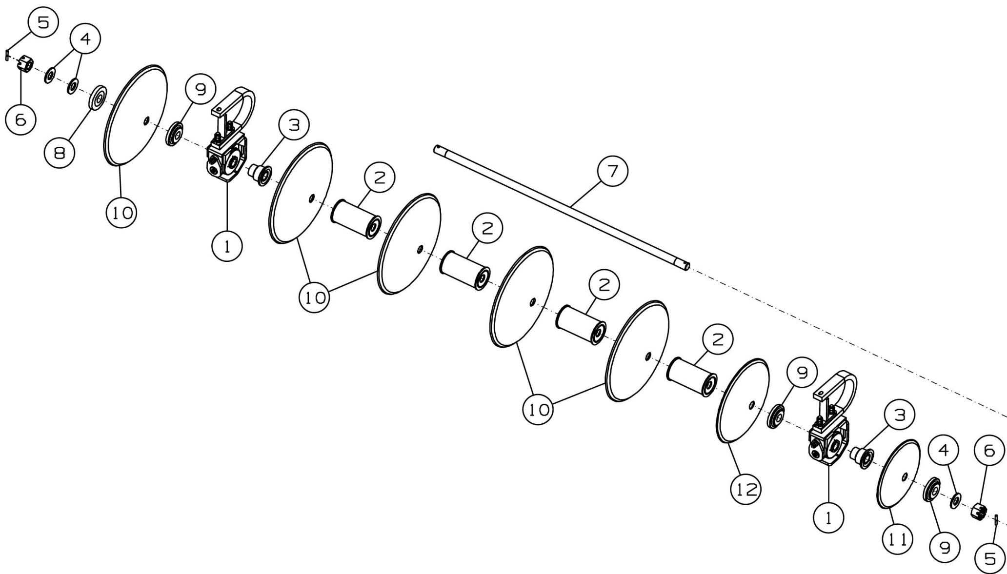
Рисунок 8 - Батарея ДХ-971.03.050А
