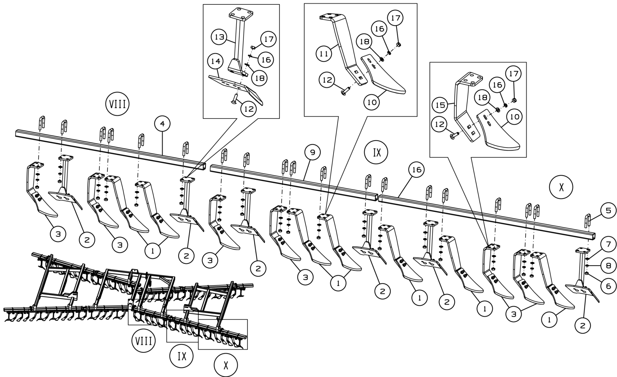
Рисунок 18 - Секция чистиков ДХ-1080.04.040Б, ДХ-1080.04.100Б и ДХ-971.04.060Б
