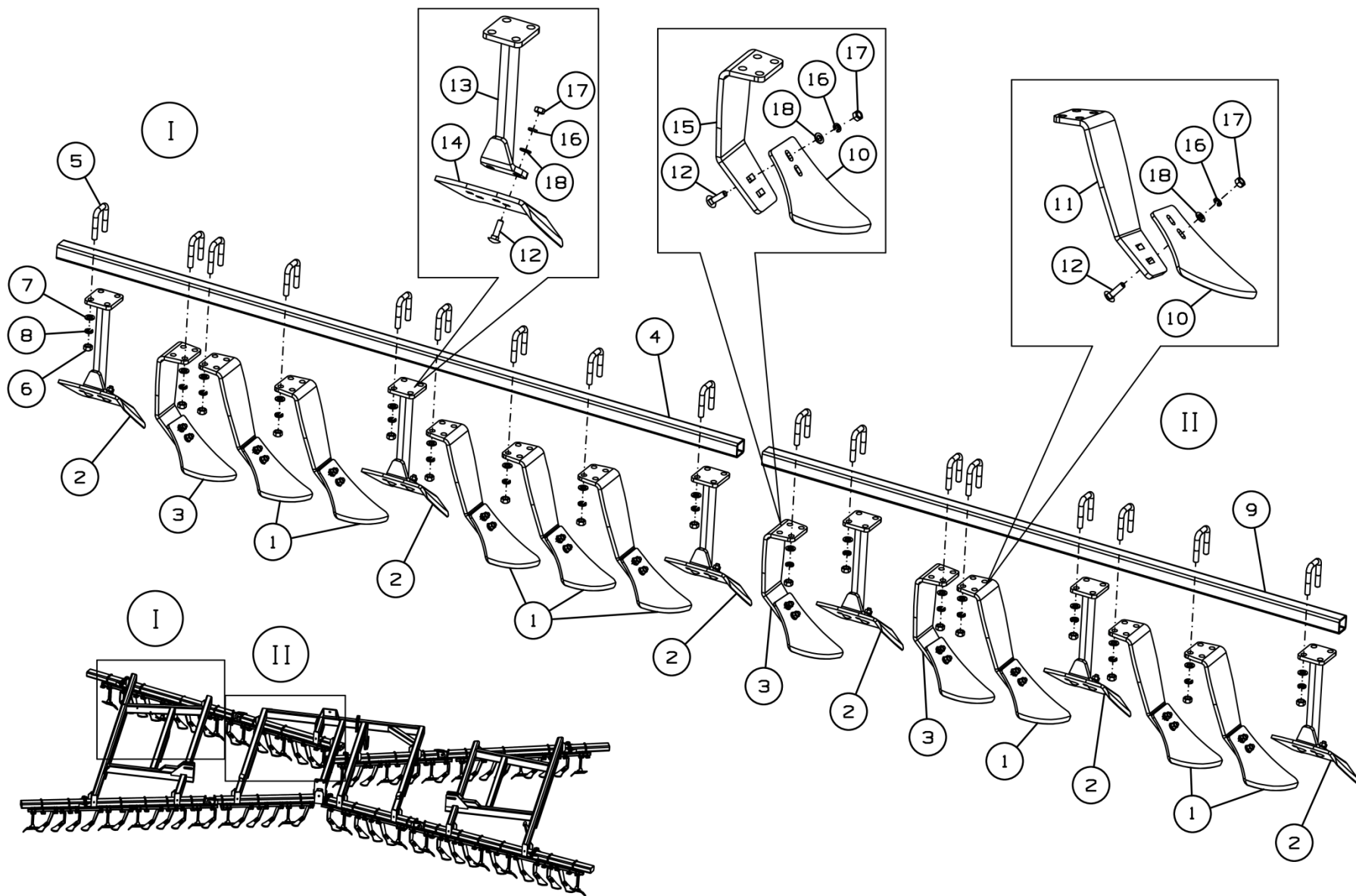
Рисунок 15 - Секция чистиков ДХ-971.04.010Б и ДХ-1080.04.010Б
