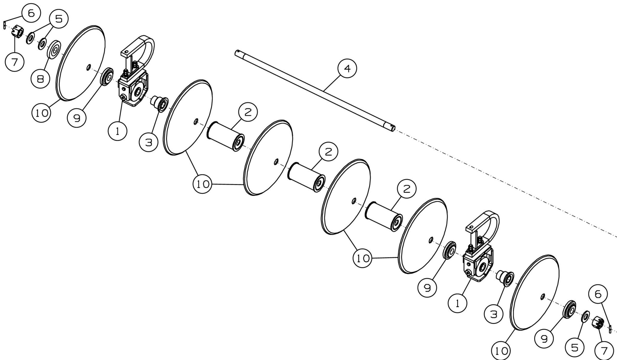
Рисунок 12 - Батарея ДХ-1080.03.040А
