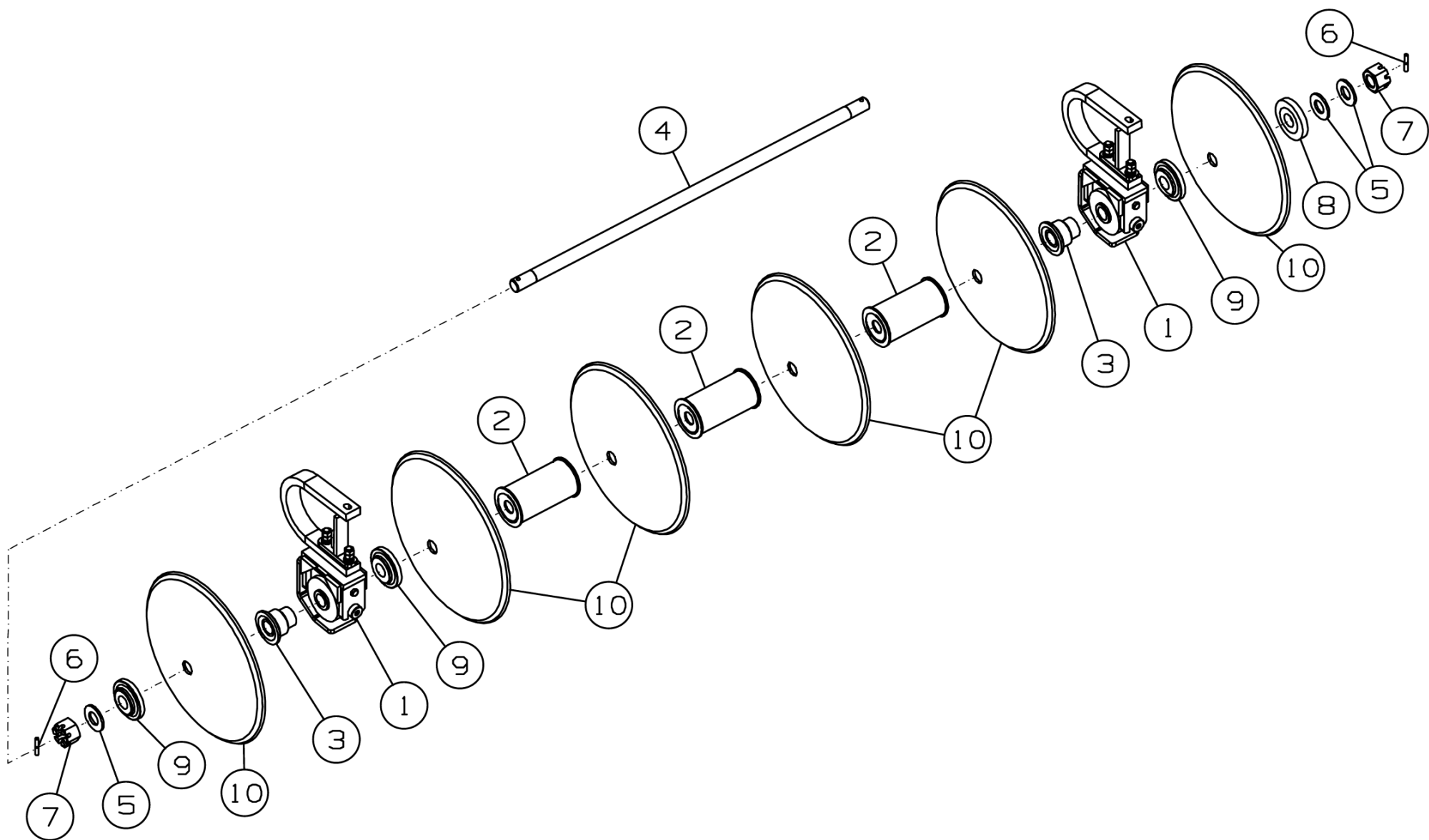
Рисунок 11 - Батарея ДХ-1080.03.030А
