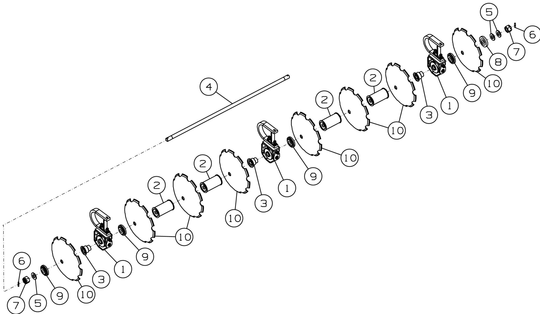
Рисунок 10 - Батарея ДХ-1080.03.020А
