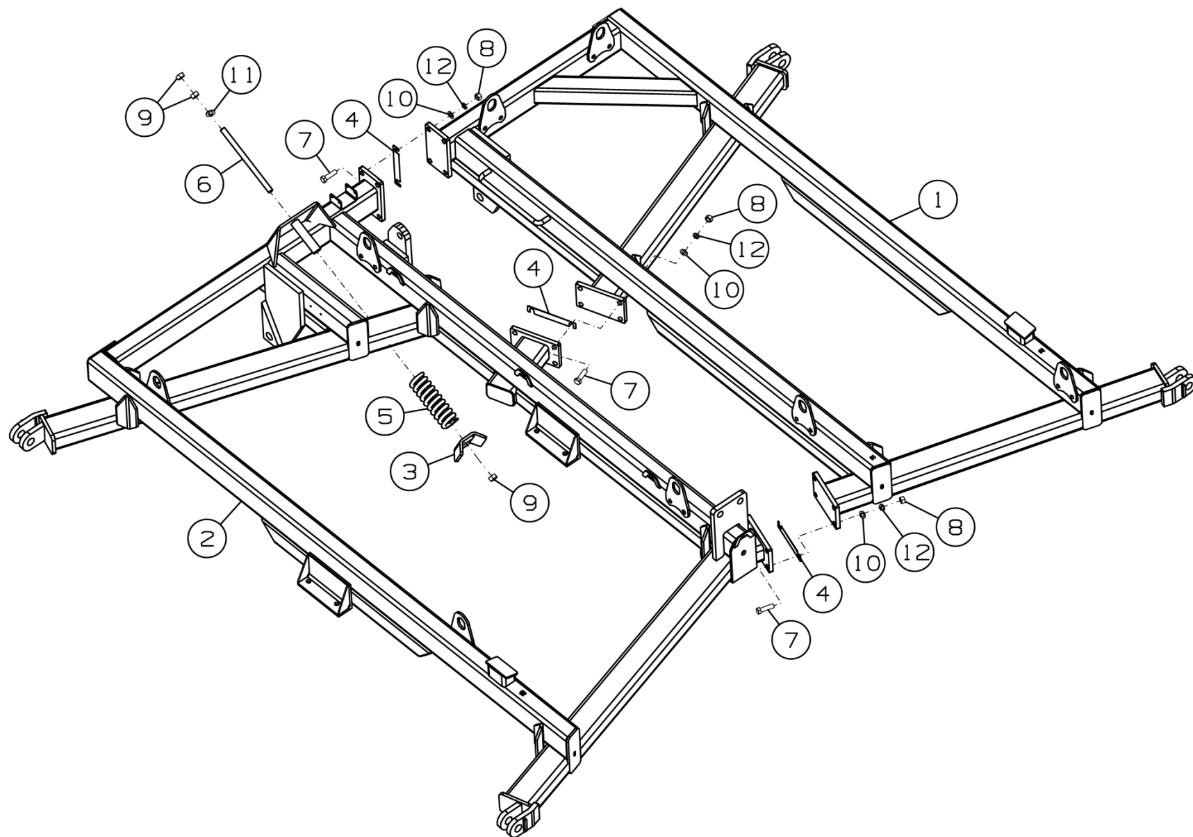
Рисунок 2 - Рама ДХ-1080.01.000
