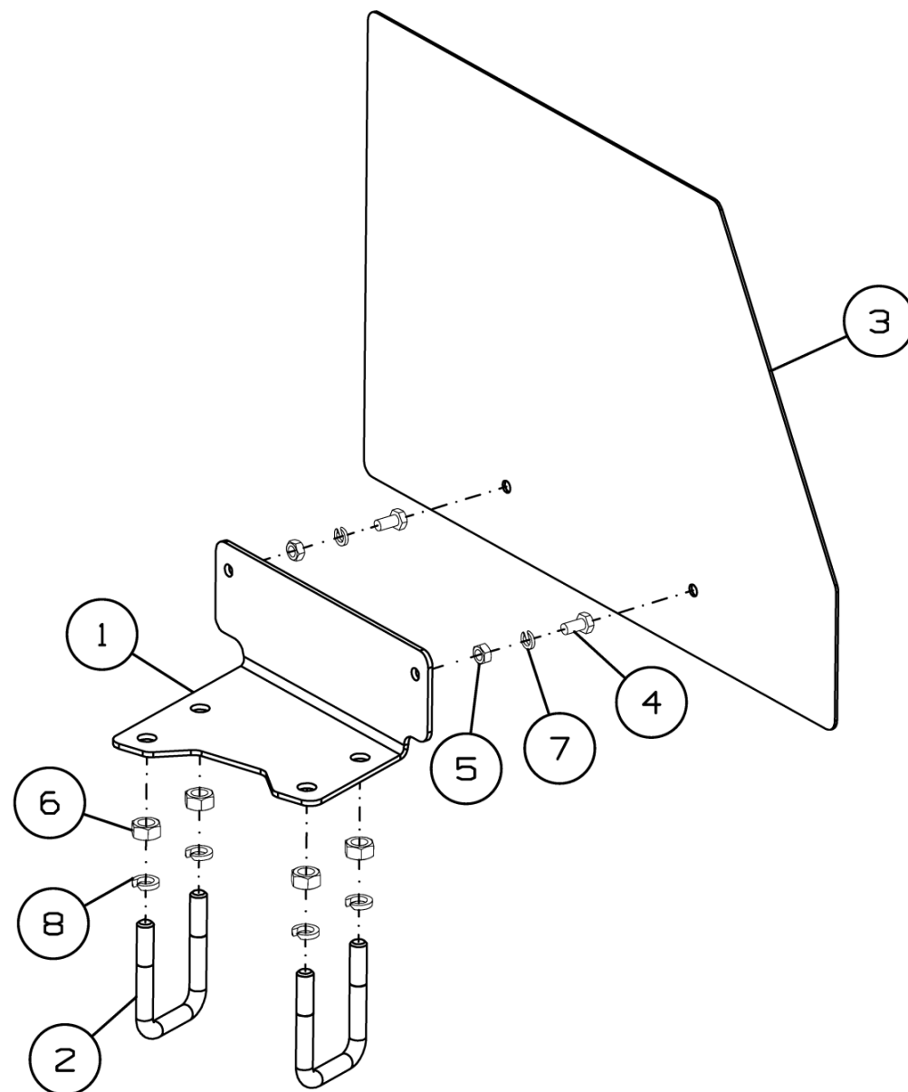
Рисунок 30 – Знак ДХ-1080.00.010
