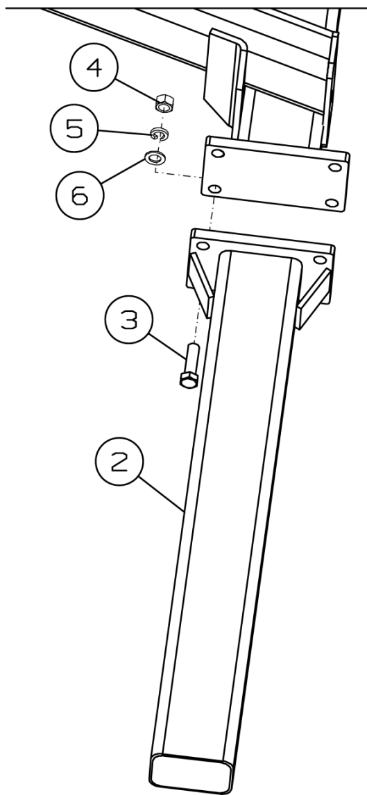
Рисунок 23 – Установка удлинителей ДХ-971.06.000
