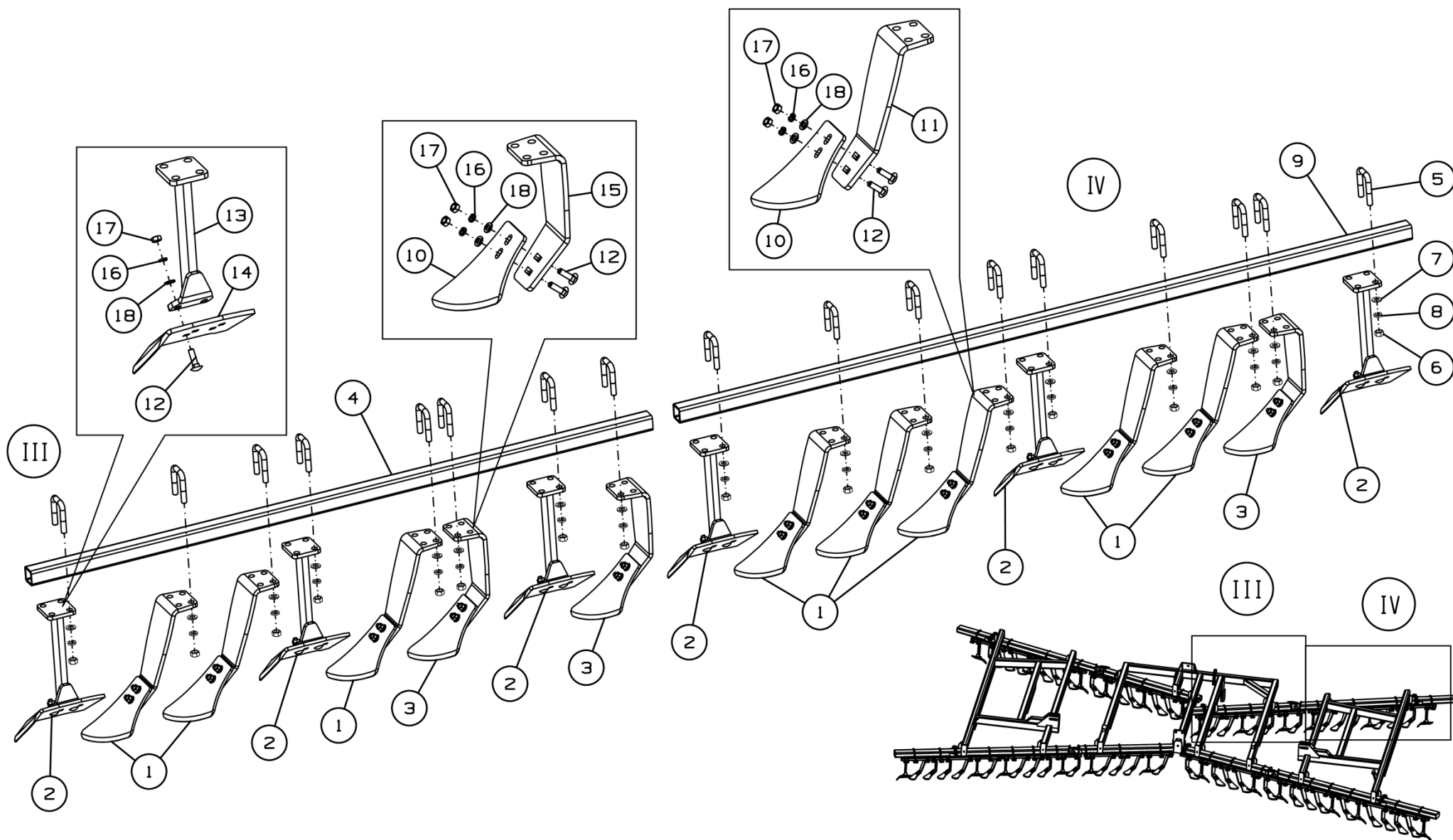
Рисунок 16 - Секция чистиков ДХ-1080.04.020Б и ДХ-971.04.020Б
