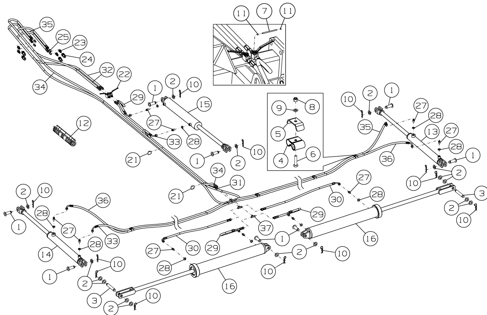
Рисунок 29 - Установка гидрооборудования ДХ-1080.12.000А-01
