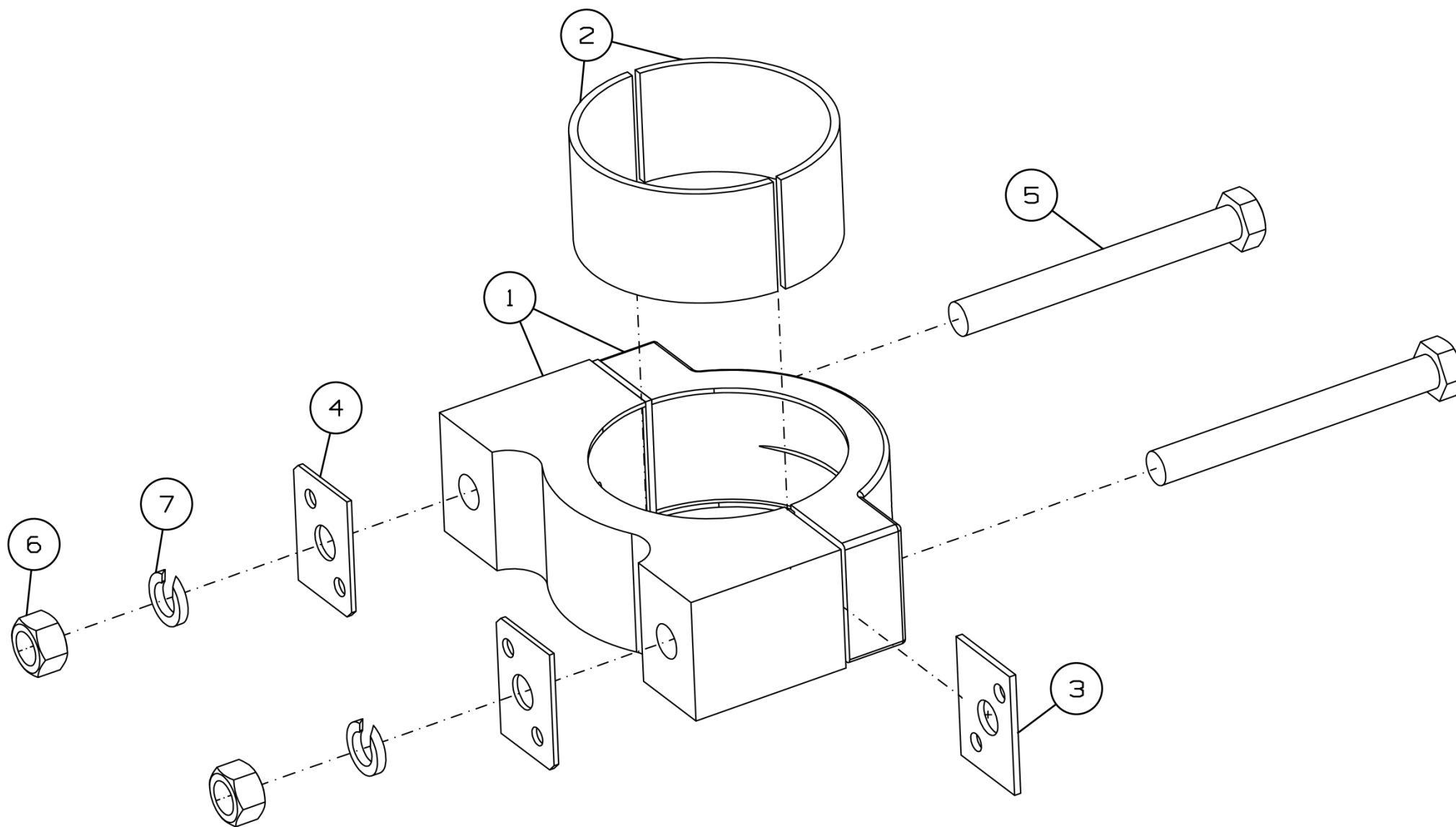
Рисунок 32 – Подшипник в сборе ДХ-1080.00.030
