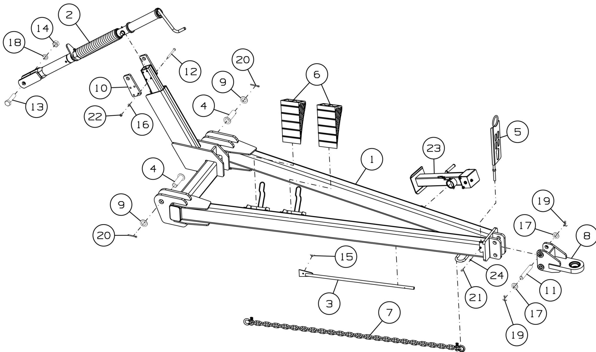
Рисунок 20 – Сница ДХ-1080.05.000Б
