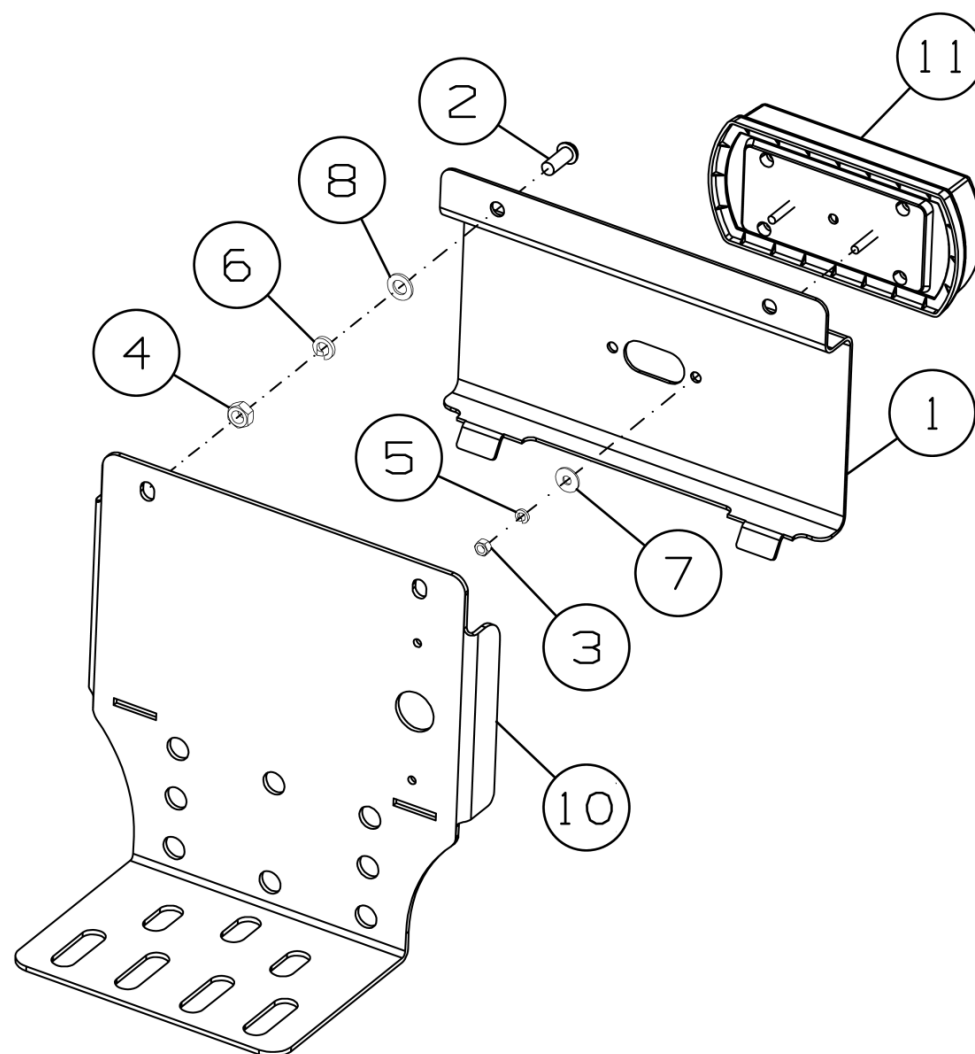
Рисунок 27 – Фонарь задний ДХ-1080.10.200 и ДХ-1080.10.200-01
