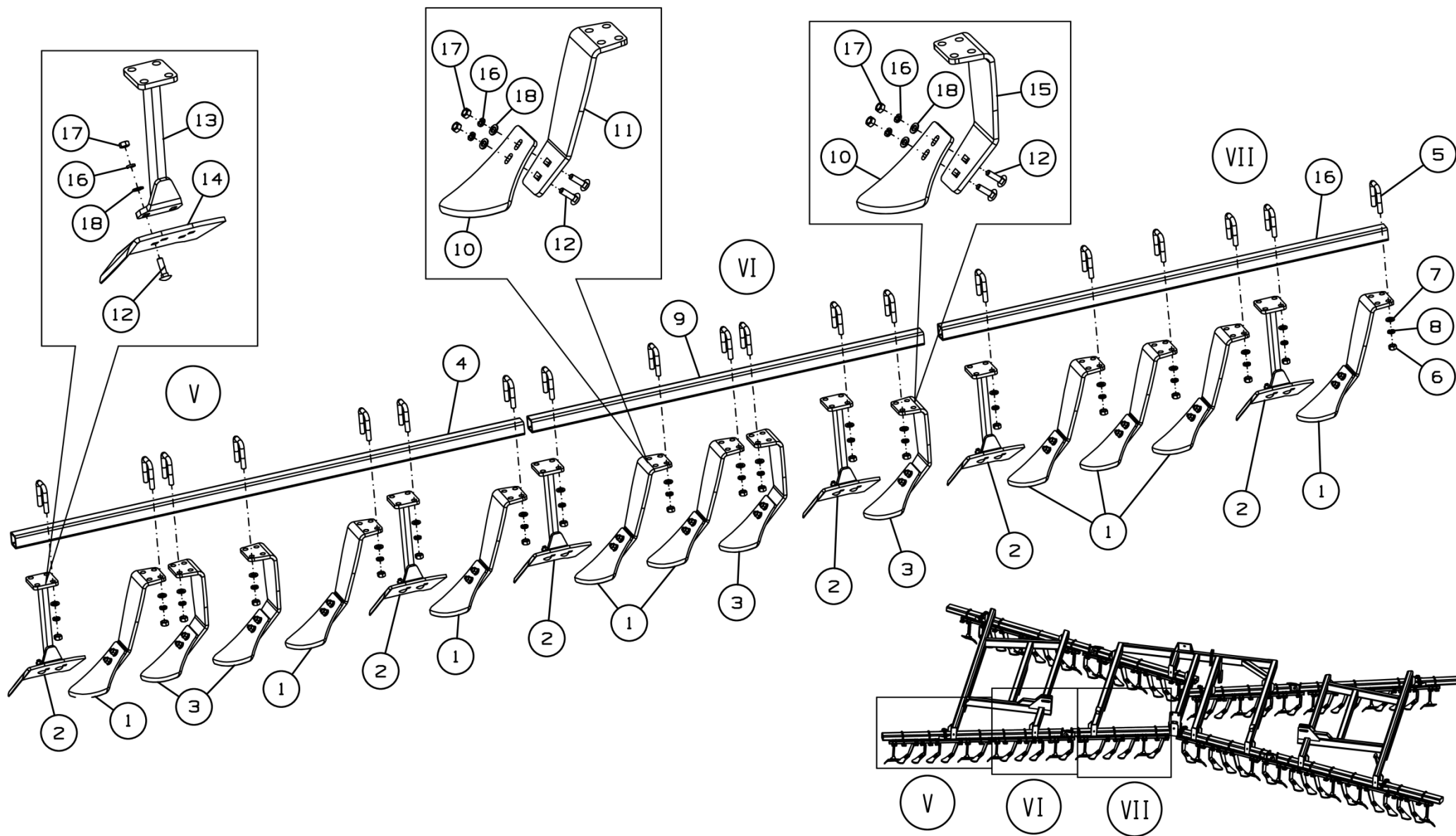
Рисунок 17 - Секция чистиков ДХ-971.04.040Б, ДХ-1080.04.090Б и ДХ-1080.04.030Б
