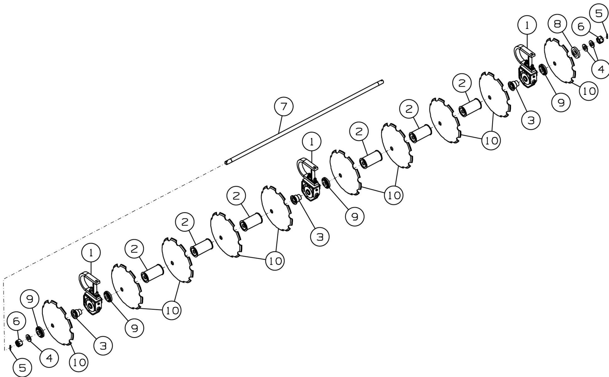
Рисунок 6 - Батарейка ДХ-971.03.020А
