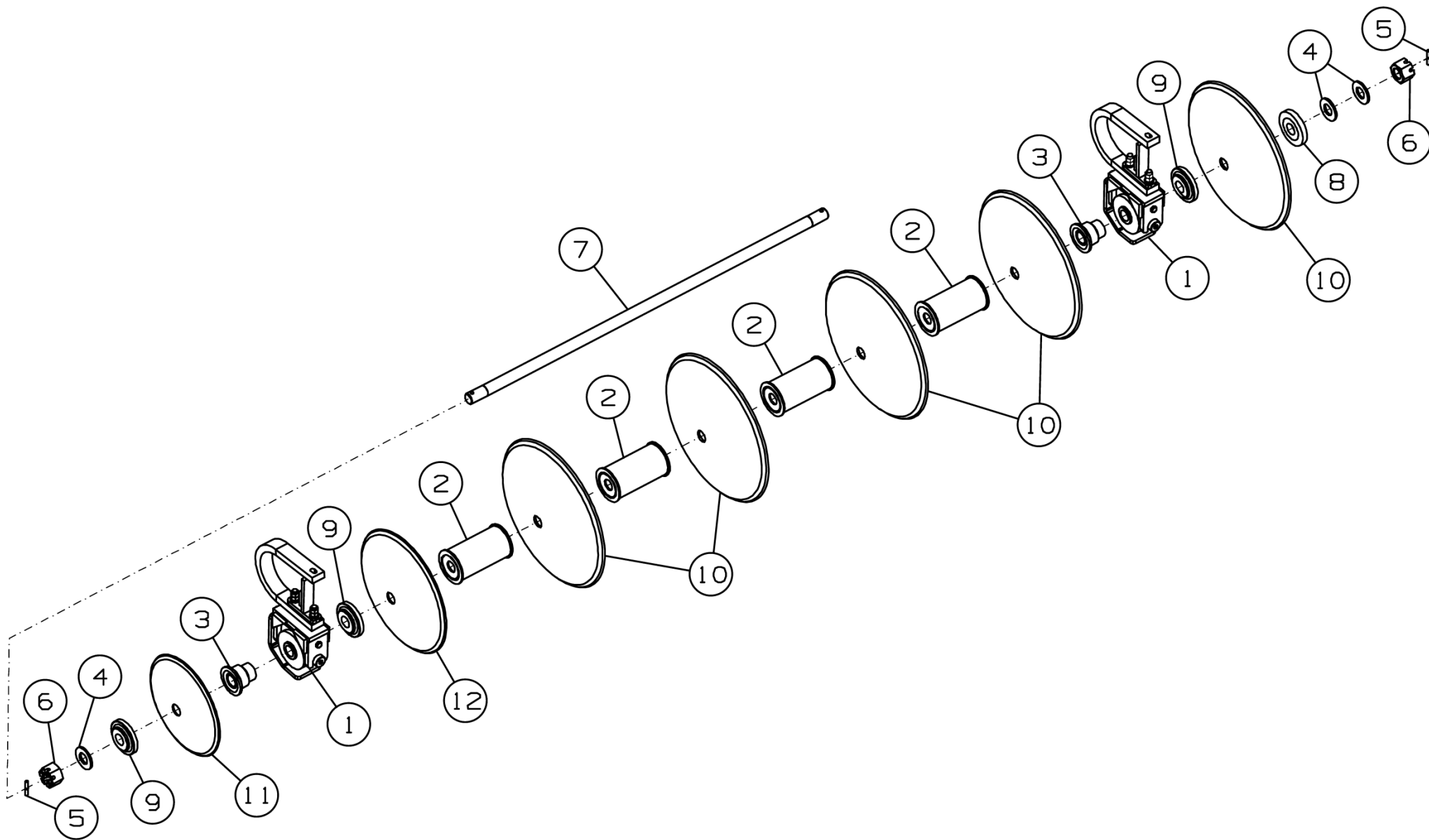
Рисунок 7 - Батарея ДХ-971.03.040А
