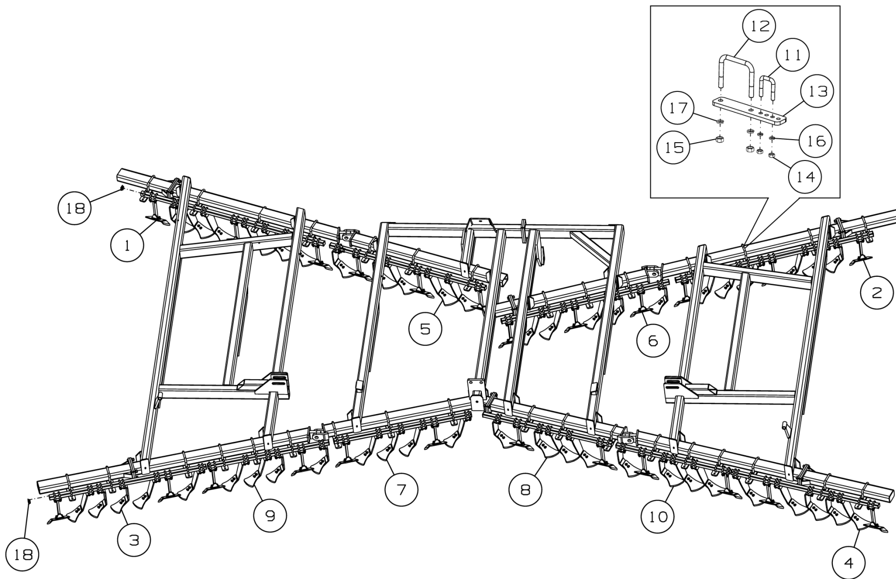
Рисунок 14 - Установка чистиков ДХ-971.04.000Б
