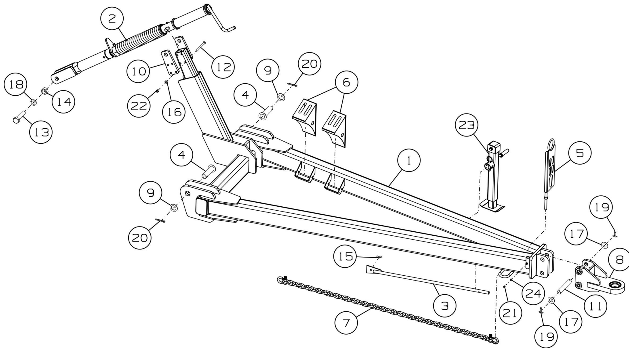
Рисунок 19 – Сница ДХ-1080.05.000А
