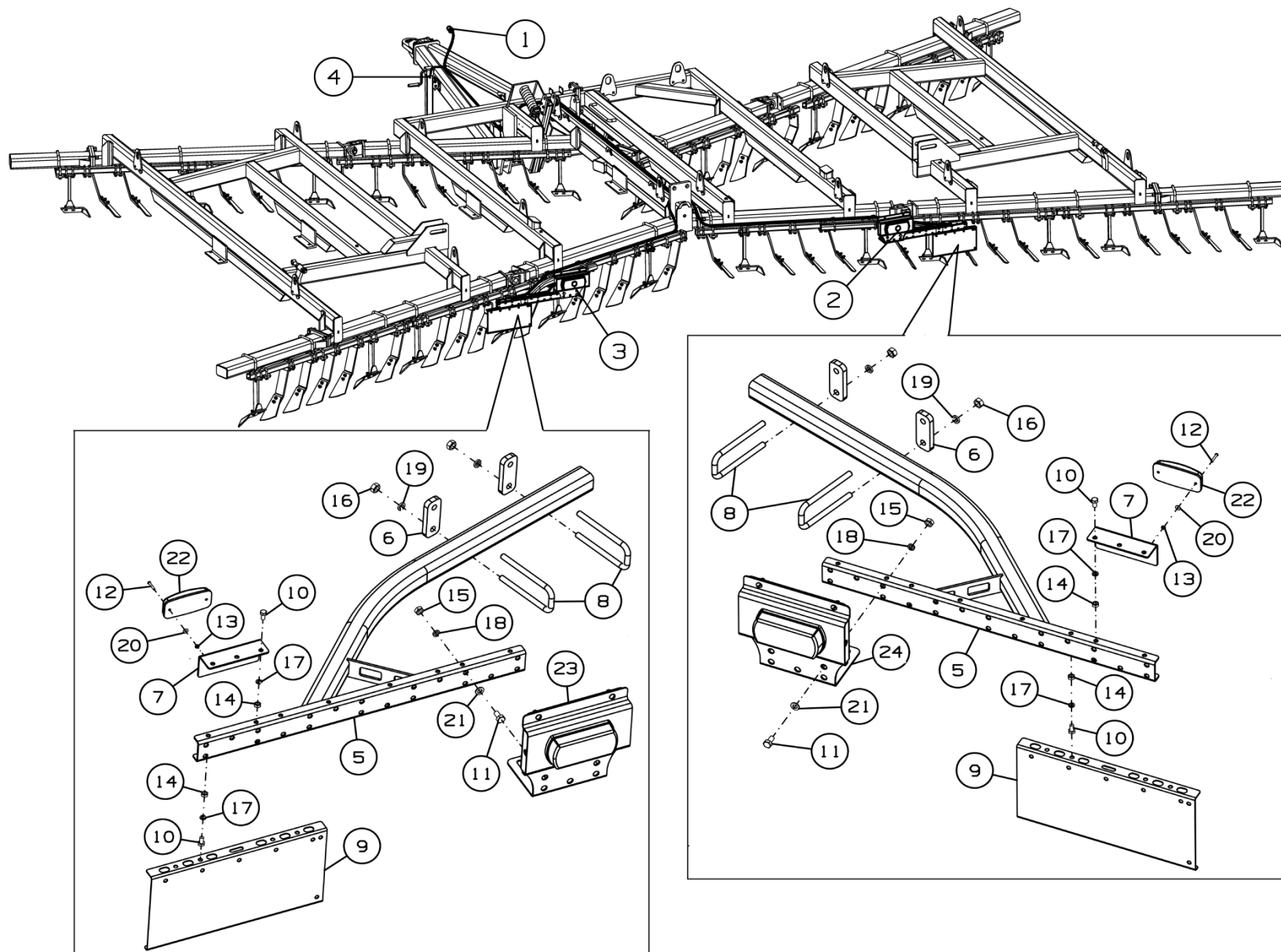
Рисунок 26 – Коммуникации электрические ДХ-1080.10.000А
