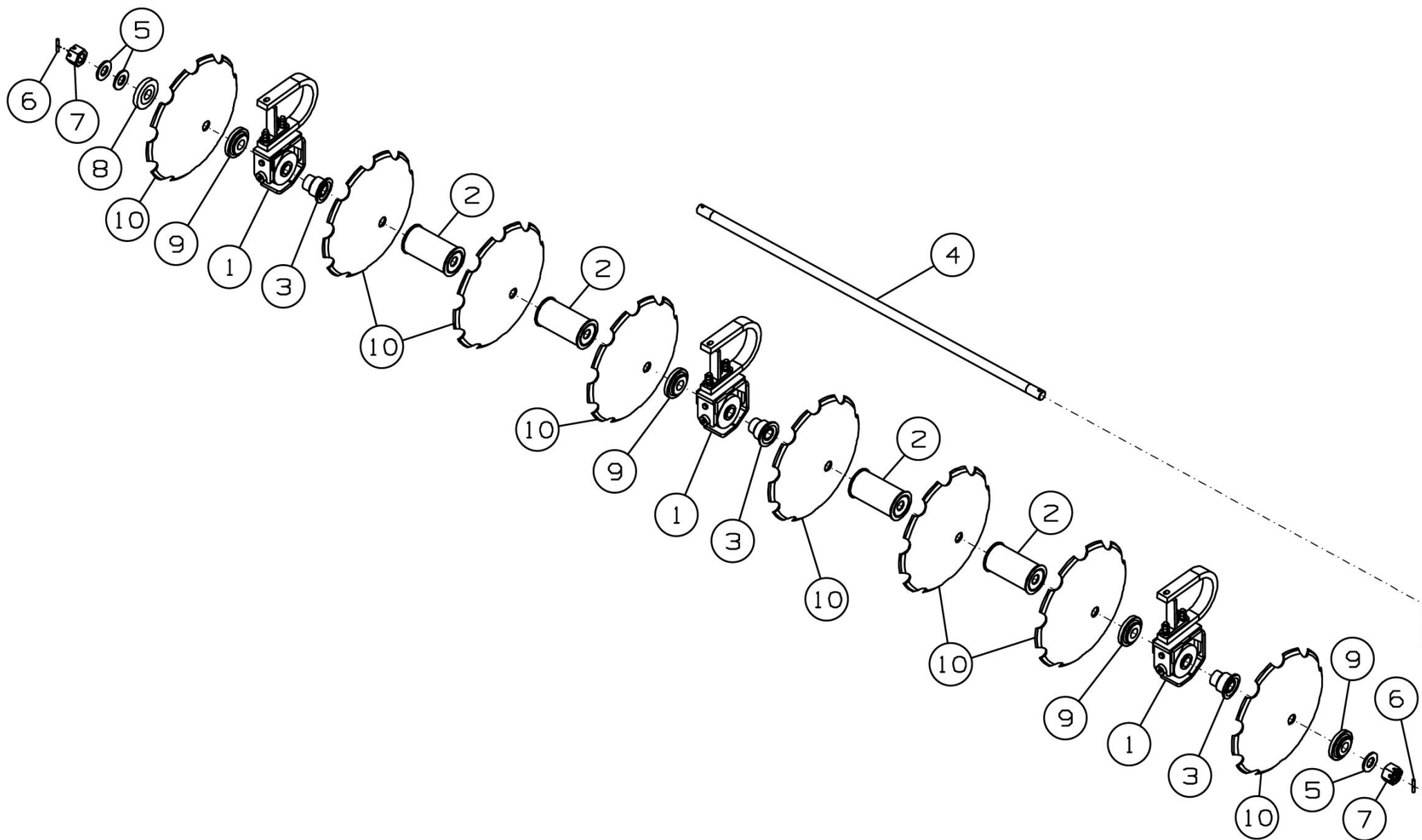
Рисунок 9 - Батарея ДХ-1080.03.010А
