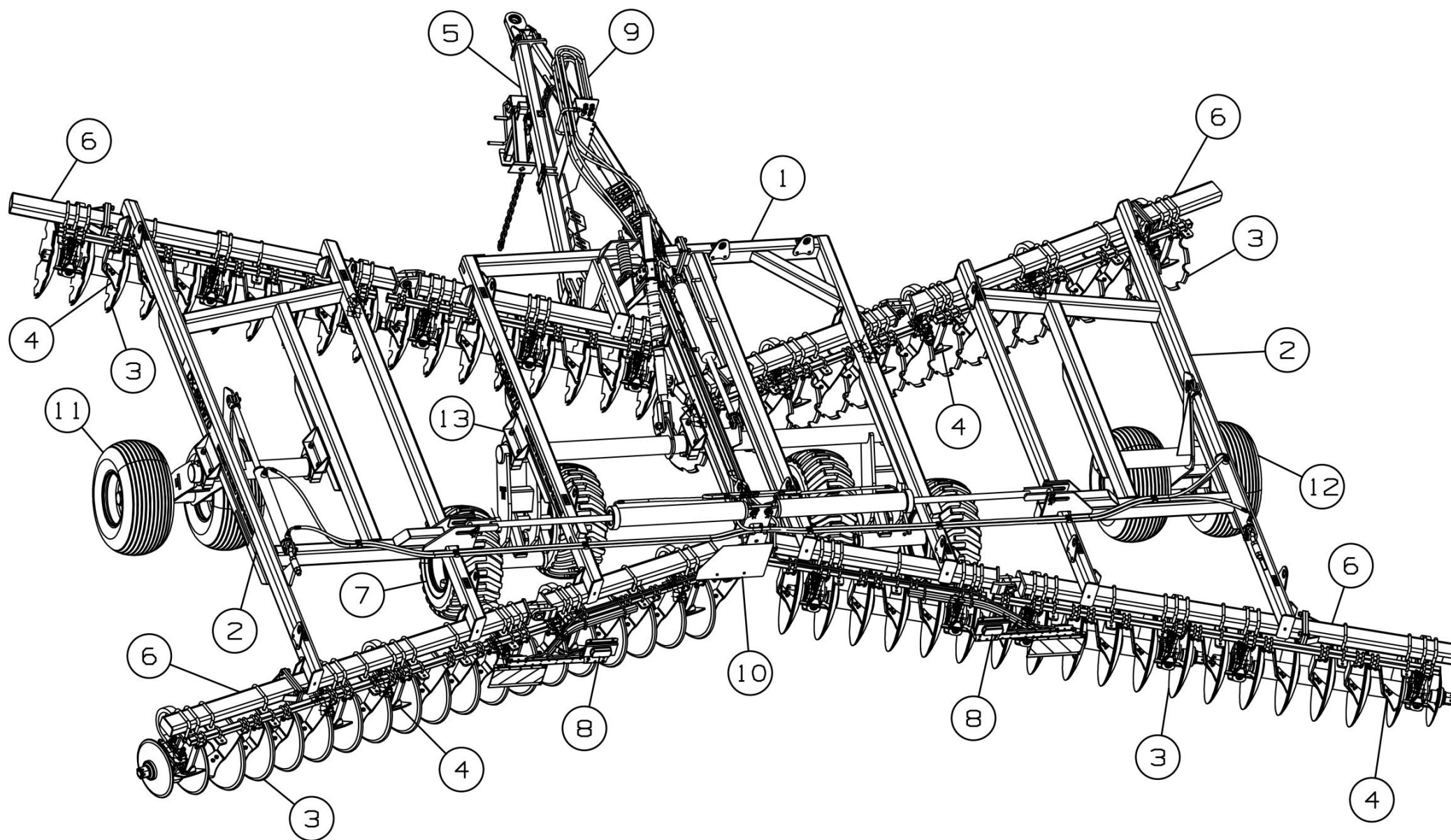
Рисунок 1 - Борона дисковая tandemная ДХ-971.00.000
